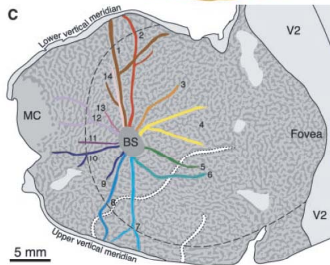
V1 (primary visual cortex)
