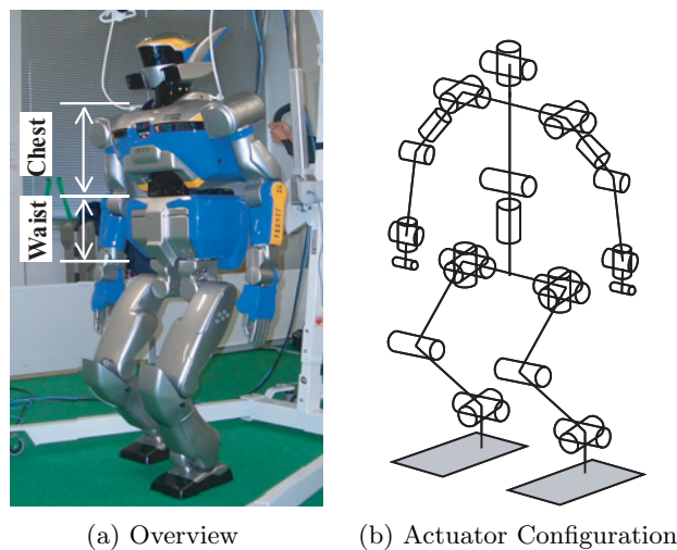
Fig. 11. Humanoid HRP-2
